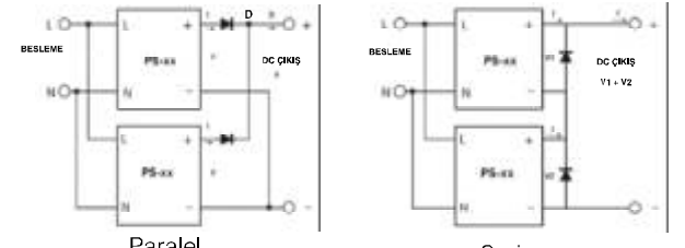
Paralel (D: ORing diyot)
